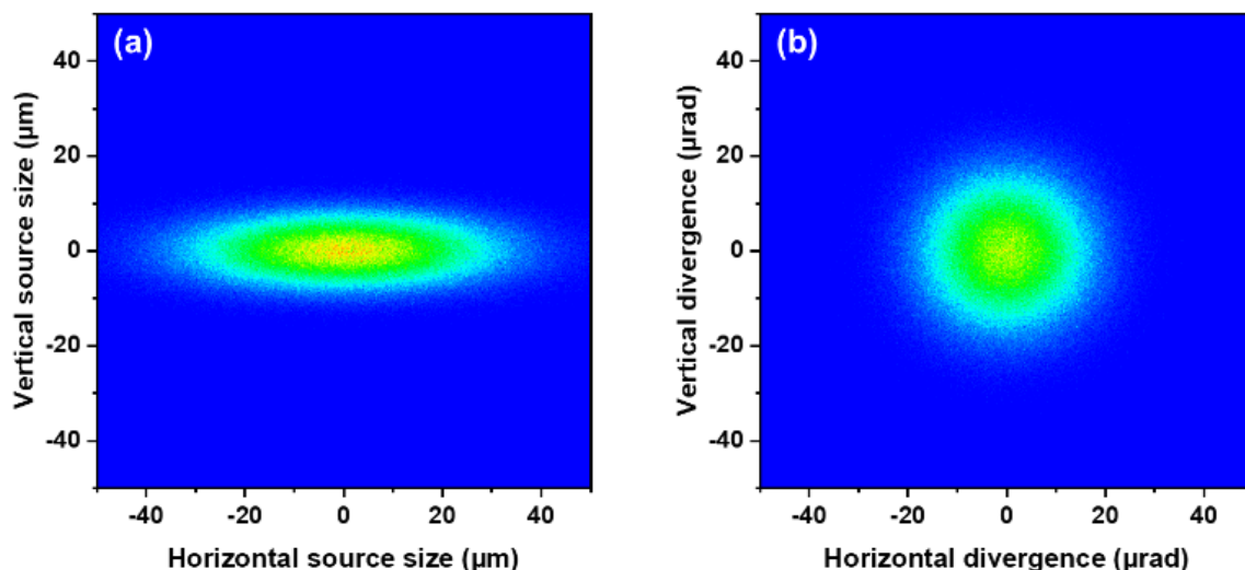
<Figure 3.2.5.4> (a) IVU22 source size, (b) divergence at 6 keV (ideal).
